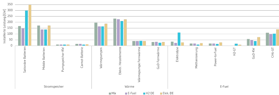
Abbildung 7.12: Installierte Leistungen der Flexibilitätsoptionen in den Szenarien Technologiemix, E-Fuels, Elektrifizierung (inländisch) und Wasserstoff (inländisch) im Jahr 2045.
